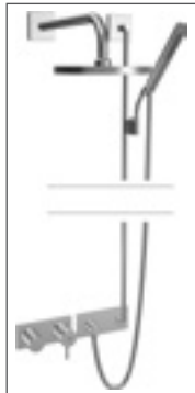
HANSAMATRIX Fertigmontage- Installationspaket 03 Einhand-Batterie, DN 15 (G 1/2)* 4487 3030 verchromt passend zu HANSASTELA, mit Wandstangen-Set, mit HANSARAIN Kopfbrause, DN 15
