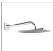
HANSAVIVA Kopfbrause, DN 15 0418 0340 verchromt Brausekopf, Messing quadratisch 250 x 250 mm Ausladung: 400 mm
