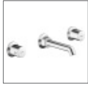
HANSADESIGNO Fertigmontageset Waschtisch-Wandbatterie für Wandeinbau, DN 15* 5106 2173 verchromt Ausladung: 200 mm
