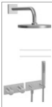
HANSAMATRIX Fertigmontage- Installationspaket 08 Thermostat-Batterie, DN 15 (G 1/2)* 4487 0080 verchromt passend zu HANSALOFT, HANSADESIGNO, HANSALIGNA, HANSASTELA, HANSARONDA, mit Brause-Set, mit HANSARAIN Kopfbrause, DN 15
