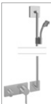
HANSAMATRIX Fertigmontage- Installationspaket 01 Einhand-Batterie, DN 15 (G 1/2)* 4487 4010 verchromt passend zu HANSALOFT, mit Ganzmetall-Wandstange 1100 mm
