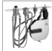
HANSA 4-Loch Universal- Wannenrand-Einbaukörper, DN 20 5304 0200 verchromt montierbar mit allen 4-Loch-Fertigmontagesets
