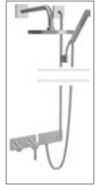
HANSAMATRIX Fertigmontage- Installationspaket 03 Einhand-Batterie, DN 15 (G 1/2)* 4487 2030 verchromt passend zu HANSARONDA, mit Wandstangen-Set, mit HANSARAIN Kopfbrause, DN 15
