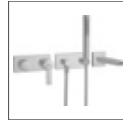
HANSAMATRIX Fertigmontage- Installationspaket 10 Einhand-Batterie, DN 15 (G 1/2)* 4487 1100 verchromt passend zu HANSALIGNA, mit Brause-Set, mit Wanneneinlauf, DN 15
