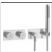
HANSAMATRIX Fertigmontage- Installationspaket 19 elektronische Thermostat- Batterie, DN 15 (G 1/2)* 4487 0190 verchromt passend zu HANSASIGNATUR, HANSALOF, HANSADESIGNO, HANSALIGNA, HANSASTELA, HANSARONDA, mit Brause-Set
