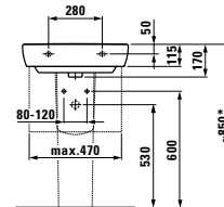
81396.7 Aufsatz-Doppelwaschtisch, Unterseite geschliffen
