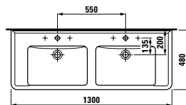
81396.7 Aufsatz-Doppelwaschtisch, Unterseite geschliffen
